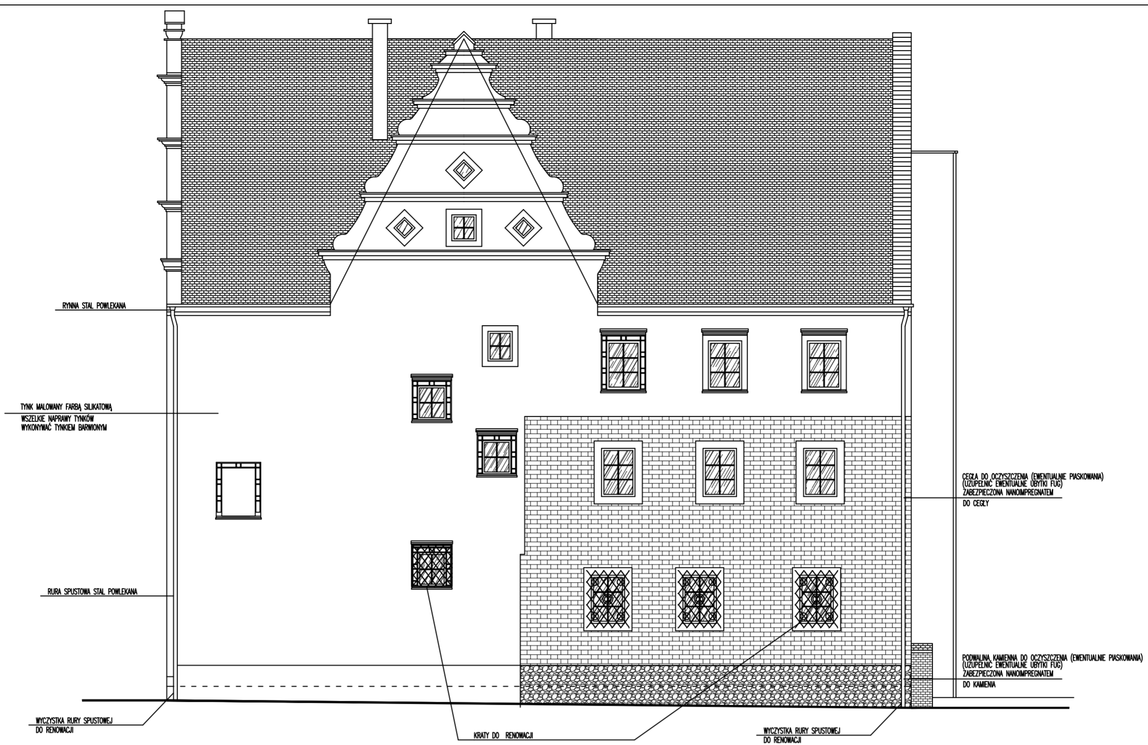
ELEVACJA PÓŁNOCNO-WSCHODNIA (BOCZNA)
